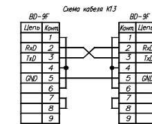
Рис. 1.3. Схема электрическая подключения блока сопряжения Топаз-306BC/07 к ПК через блок сопряжения "Топаз-119-5М".
