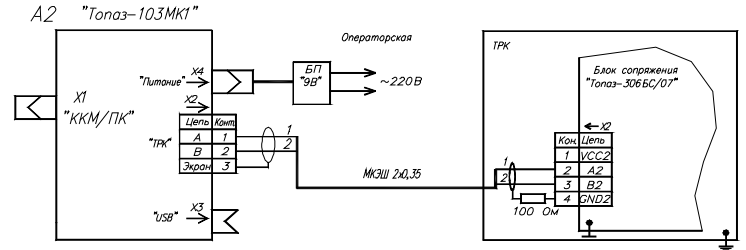
Рис. 1.2. Схема электрическая подключения блока сопряжения Топаз-306BC/07 к контроллеру "Топаз-103МК1".
