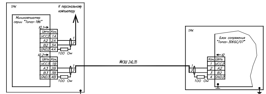
Рис. 1.4. Схема электрическая подключения блока сопряжения Топаз-306BC/07 к миникомпьютеру серии "Топаз-186".
